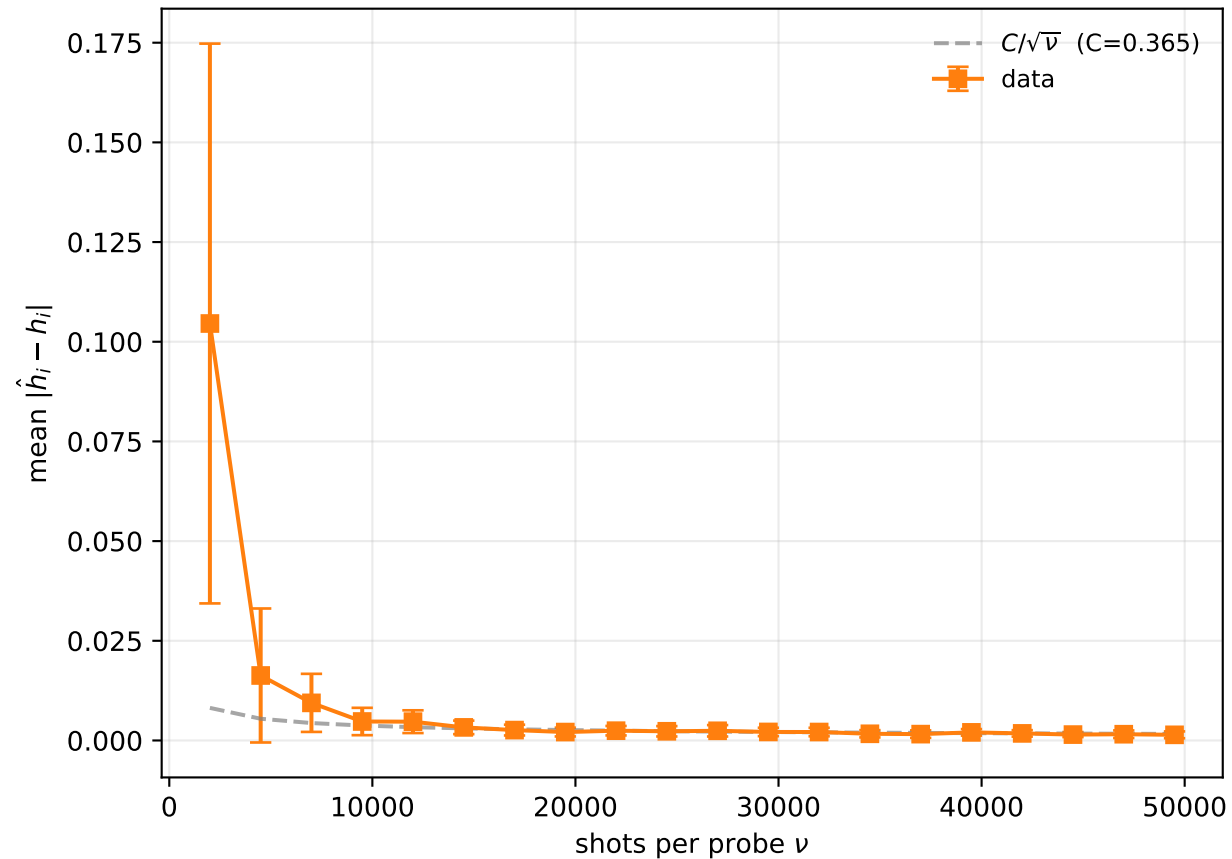
TFIM, n=10 , probes=1000
