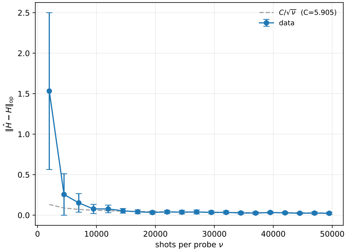
TFIM, n=10 , probes=1000
